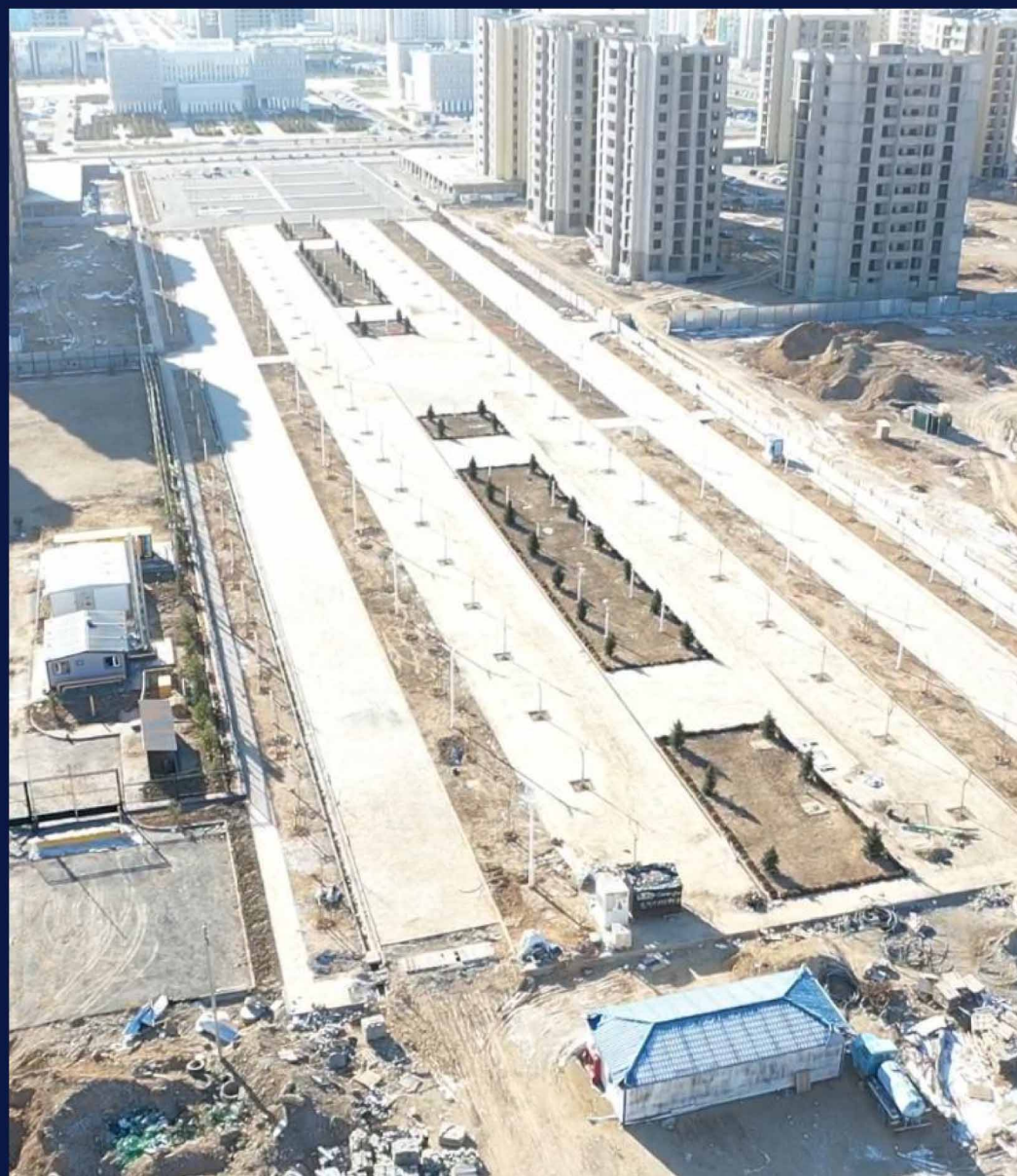
Земляные работы
